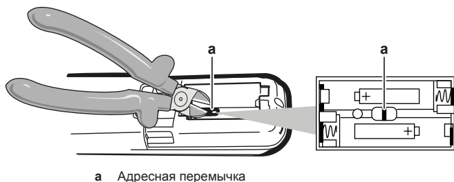
а Адресная перемычка
